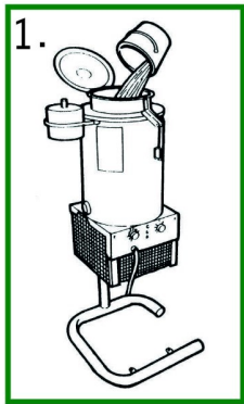
1. 置入回收袋倒入廢溶劑。
